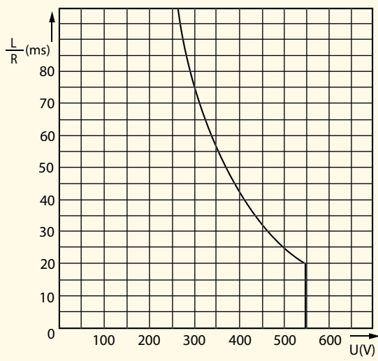
Dane dla wykonań DC 22X58 URD
