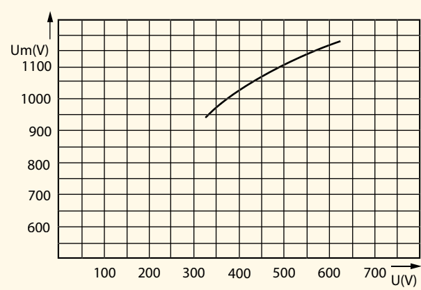
Maksymalne napięcie łukowe 22X58 URD
