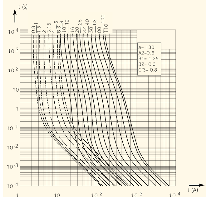
Charakterystyka czasowo-prądowa
