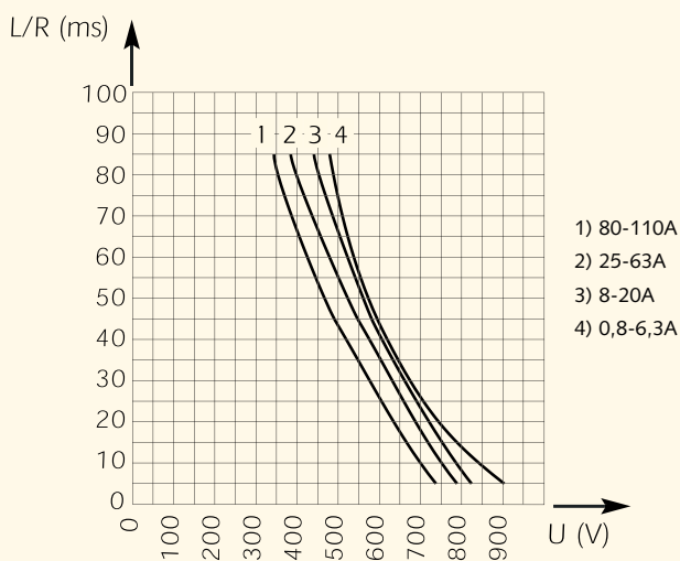
Charakterystyka L/R
